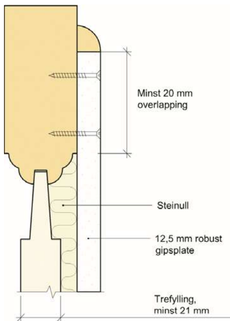
Figur 3-7 Ensidig tildekking på dørblad når trepanelet er minst 21 mm. Løsningen er basert på [4].
