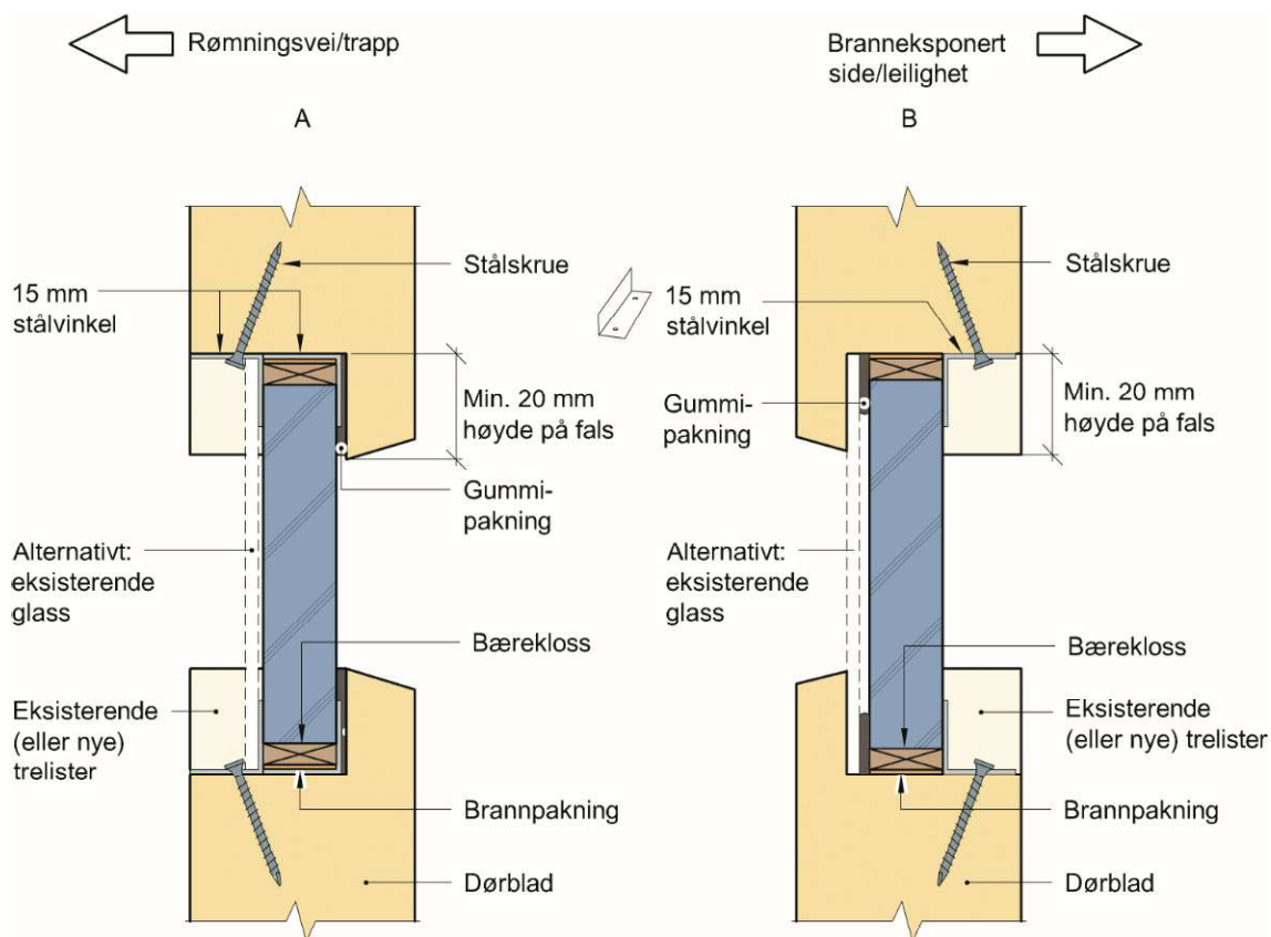
Figur 3-1 Mulige måter å montere brannklassifisert glass på
